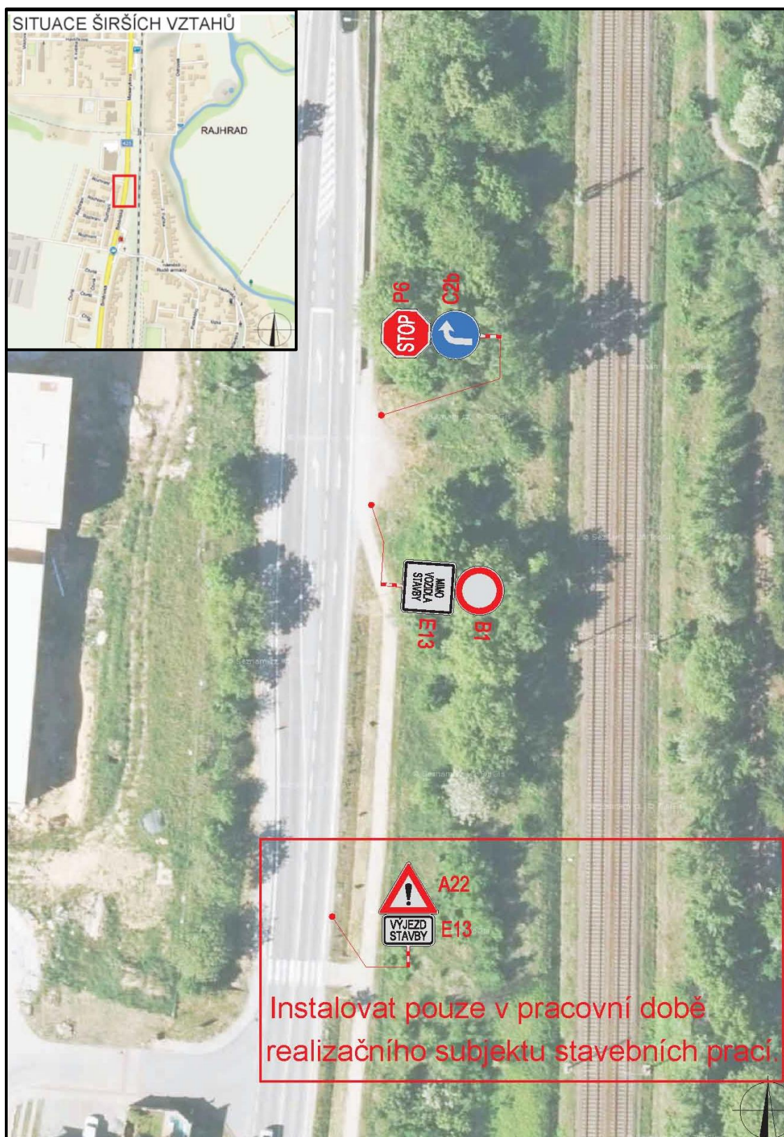
Obr. 1 – Situace dopravního značení
