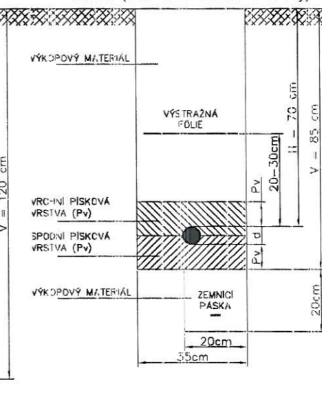
obr. 1 – ULOŽENÍ VE VOLNÉM TERÉNU TERÉN (bez mechanické ochrany)
