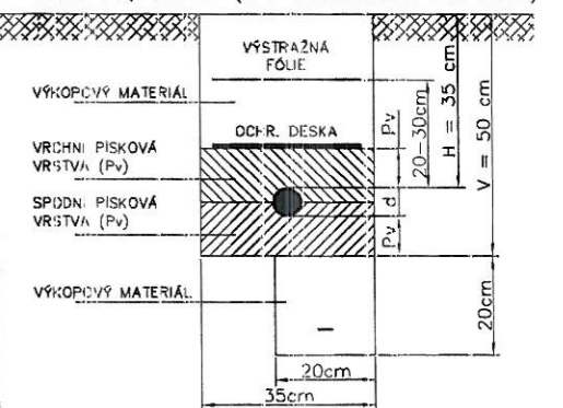
obr. 3 – ULCŽENÍ V CHODNIKU CHODNÍK, TERÉN (s mechanickou ochranou)
