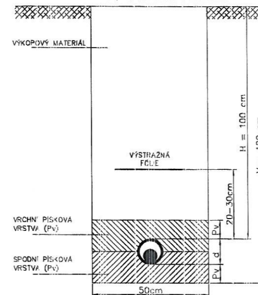
obr. 1 – ULOŽENÍ S CHRÁNIČKOU VOZOVKA, KRAJNICE VOZOVKY
