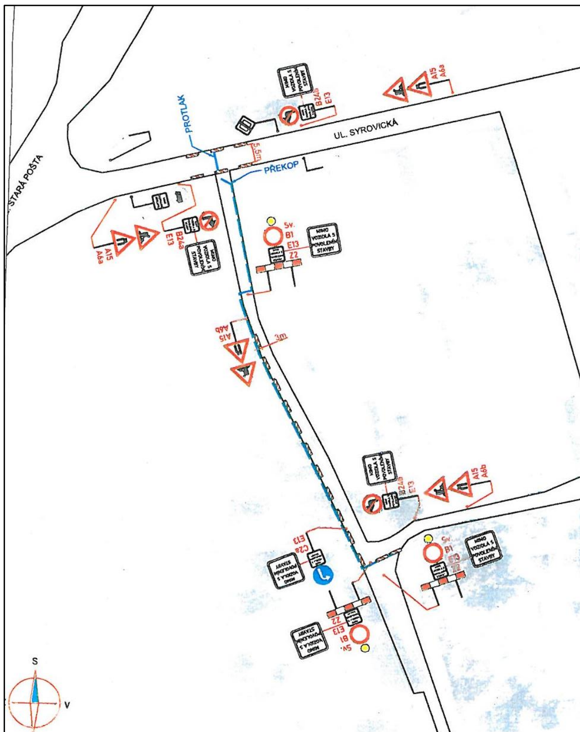
Obr. 1 – situace dopravního značení
