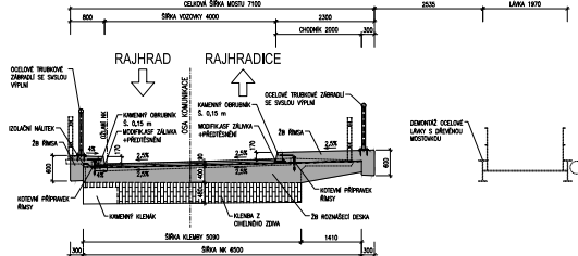
Doporučená varianta 2, příčný řez
