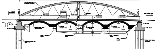
Nedoporučená varianta C, podélný řez
